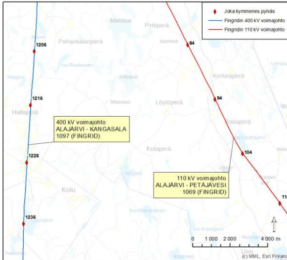
Kuva 1. Fingridin voimajohdot.
